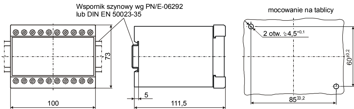
Rys. 2. Wymiary gabarytowo-montażowe przetworników mocy
