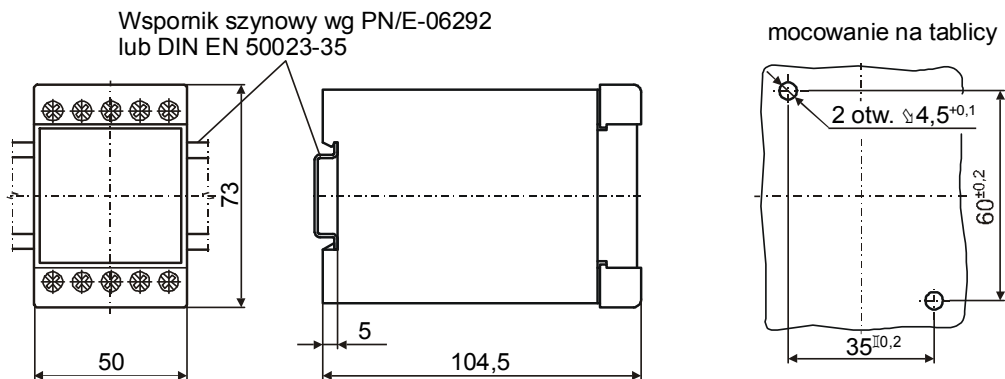
Rys. 1. Wymiary gabarytowo-montażowe przetworników prądu i napięcia
